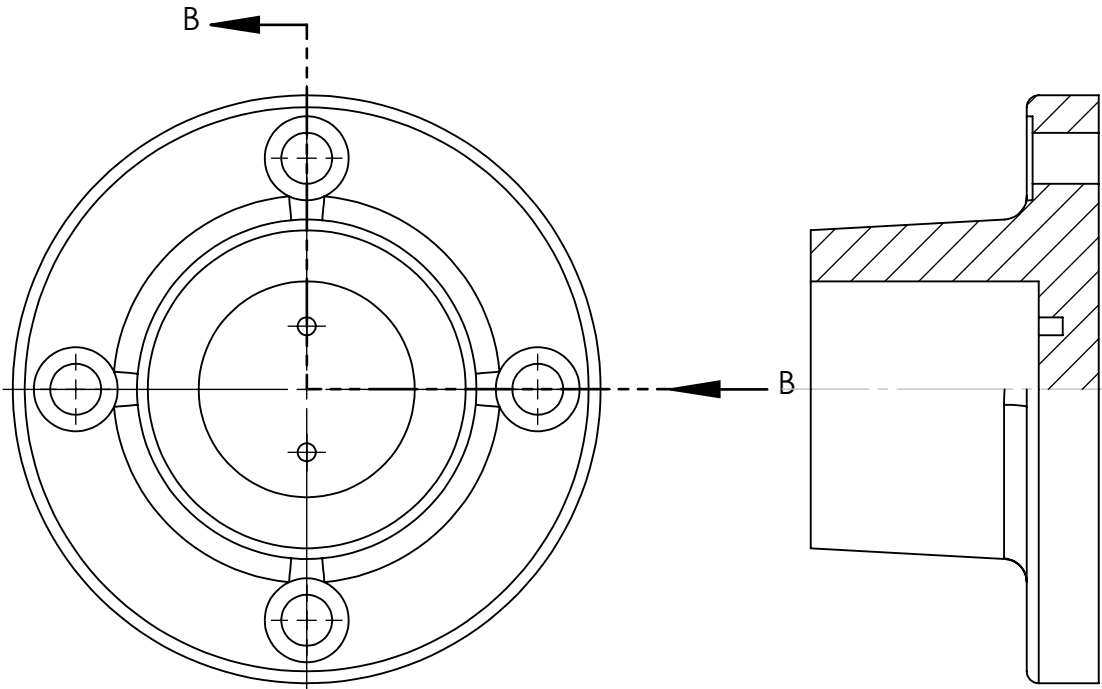
SECTION B-B SCALE 1 : 2
